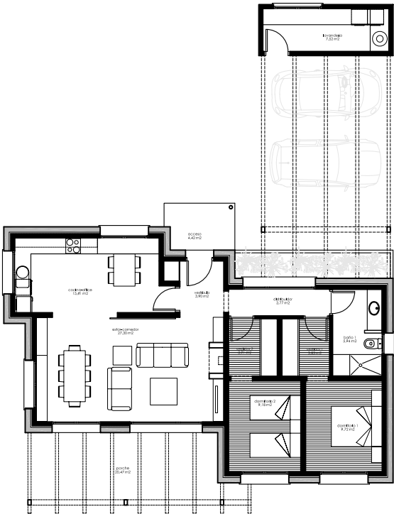
planta baja
