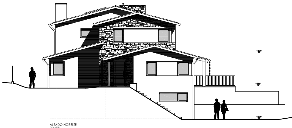
ALZADO NORESTE ESCALA 1/200
