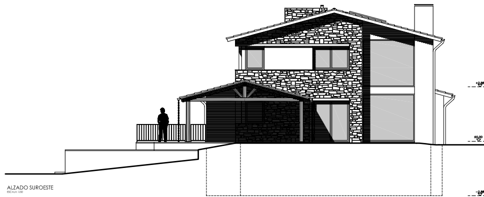
ALZADO SUROESTE ESCALA 1/200
