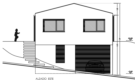
ALZADO ESTE
