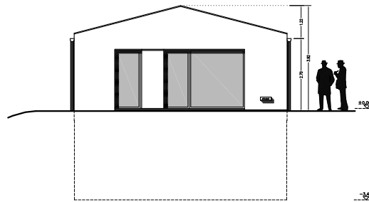
ALZADO OESTE
