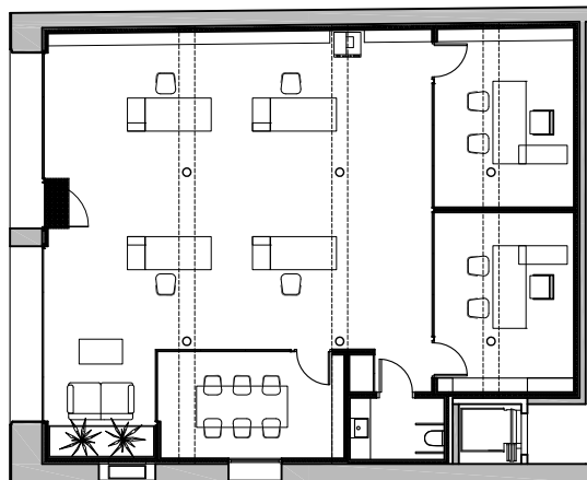
PLANTA ESCALA 1/200
