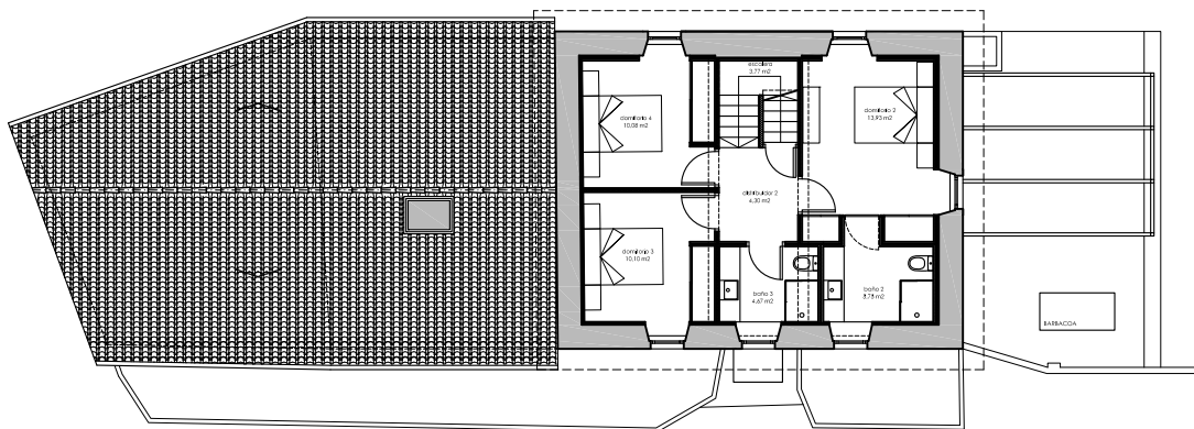
PLANTA PRIMERA ESTADO REFORMADO
