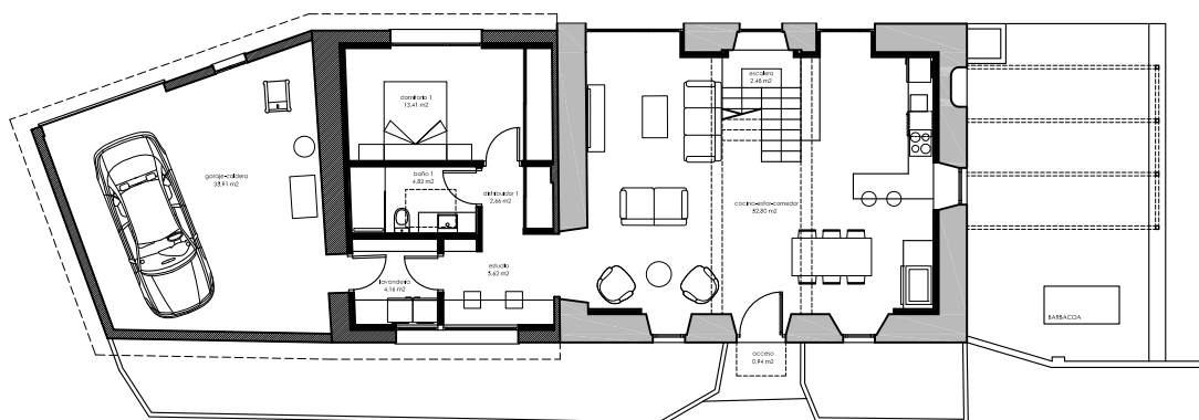
PLANTA BAJA ESTADO REFORMADO
