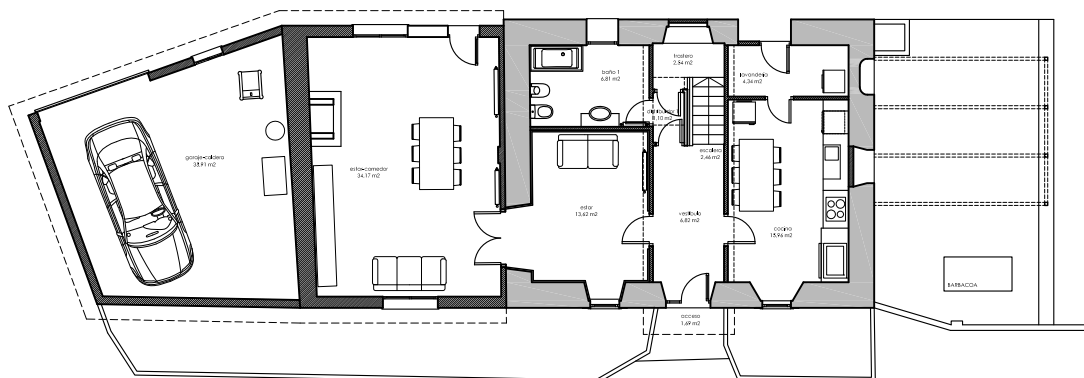
PLANTA BAJA ESTADO ACTUAL
