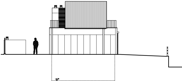
ALZADO NORTE
